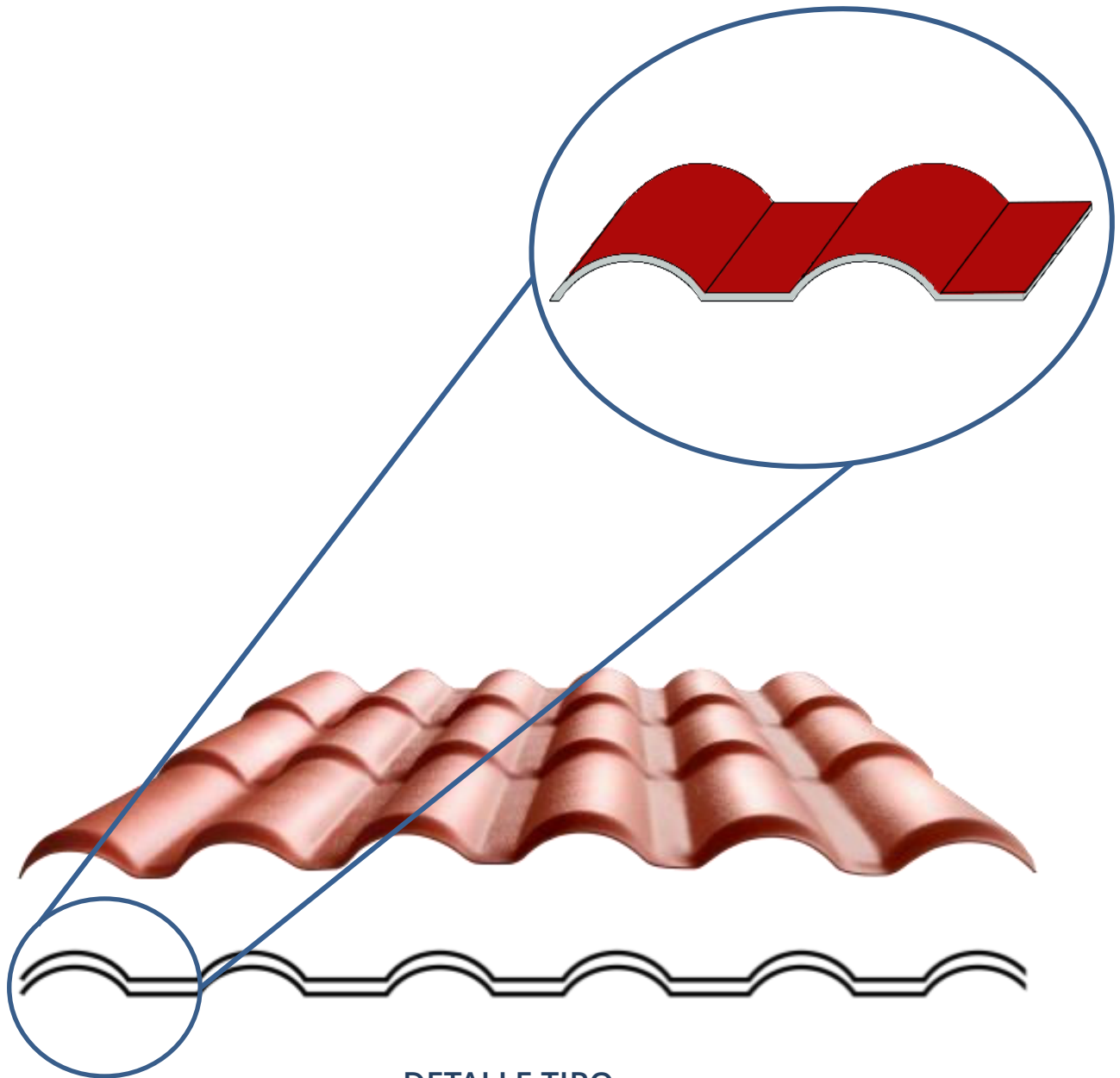
DETALLE TIPO.
